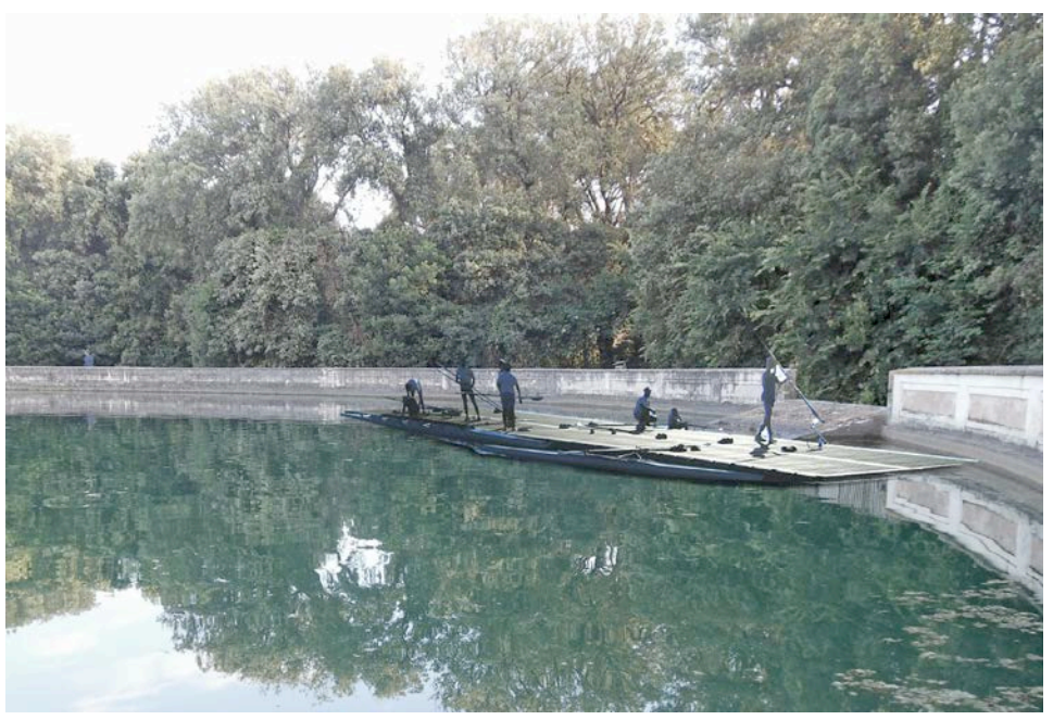
posizionamento del pontile galleggiante sulla peschiera
